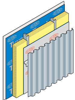
Fig. 9 Metal clad
