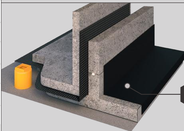
GP® TITANTANK
